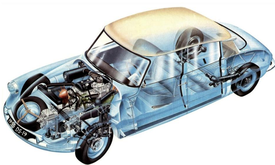
schema funzionale delle sospensioni idropneumatiche della Citroen DS 19 - 1955
