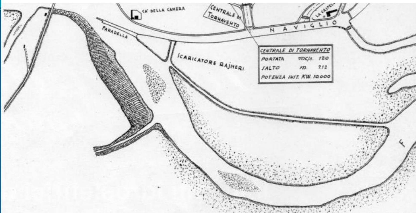
Planimetria dell'impianto di Tornaento originale, da " https://cpcontainer.weebly.com/centrali-idroelettriche.html? "
