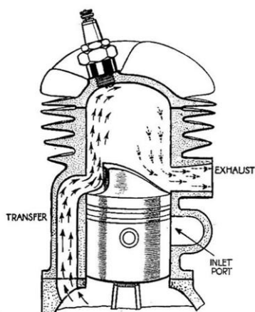
Spaccato di un motore a due tempi, privo di valvole
