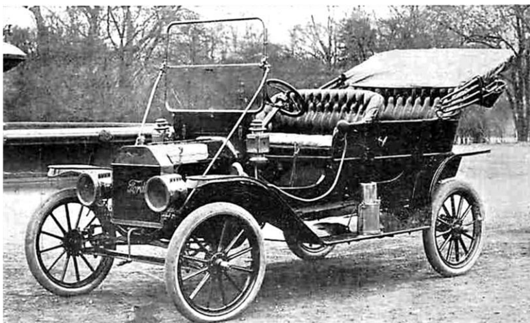
Ford T in una delle prime serie, priva delle porte anteriori - 1910
